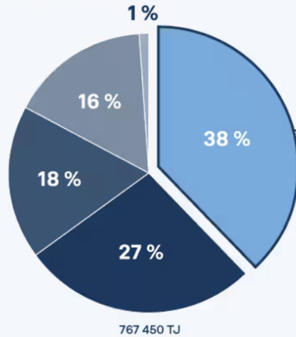
Endenergieverbrauch 2023
