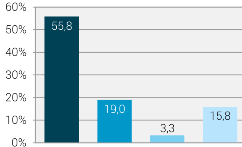
Zunahme 1979/85–2013/18
