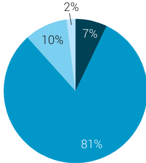
Struktur 2013/18
